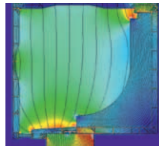
Raspored izoterma
